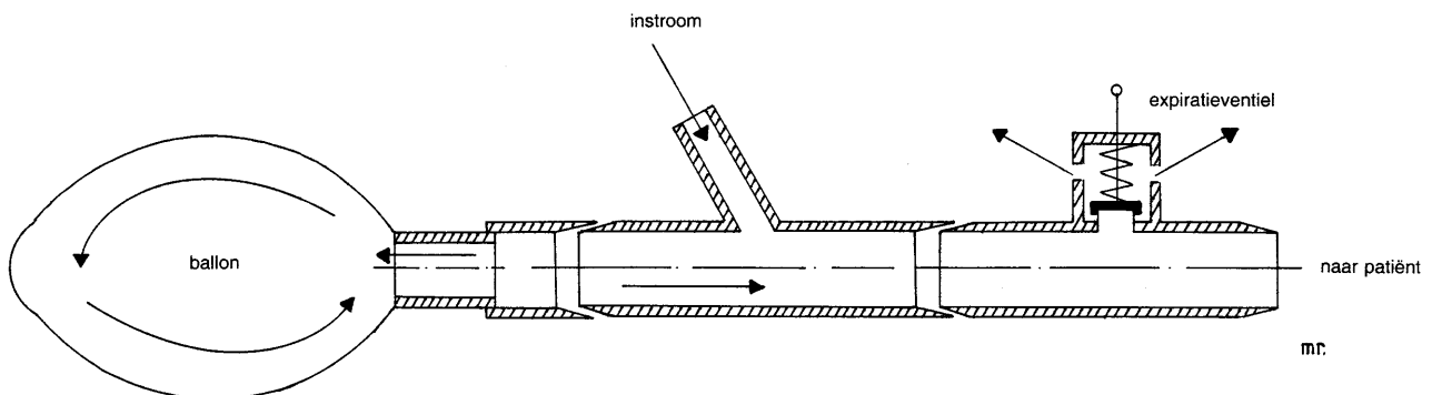
Tekening 2. Apparatuur met een slappe ballon of Jackson Rees-systeem ("Watersset") Bij deze systemen stroomt expiratielucht terug in de zak of ballon, die daardoor besmet kan raken tijdens het gebruik. De uitade-
