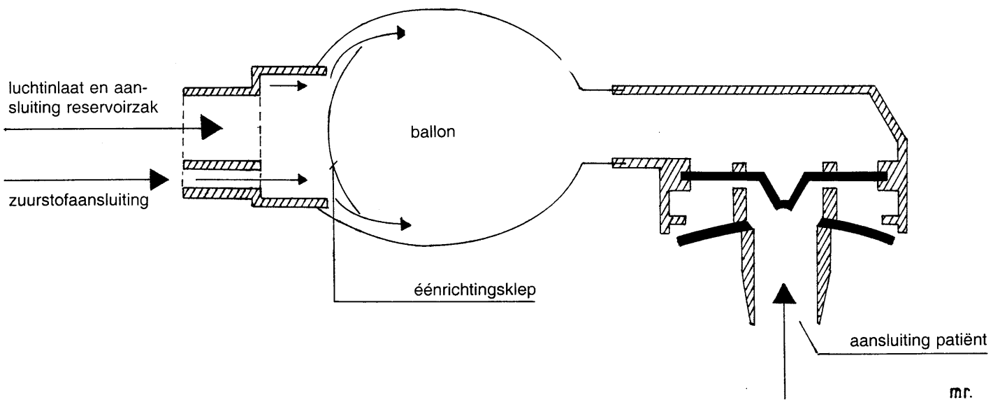
Tekening 1. Zelfontplooiende ballon (bijvoorbeeld AMBU of Laerdalset) Bij dit systeem verdwijnt de expiratielucht via het kleppensysteem en kan niet terugstromen in de ballon.
